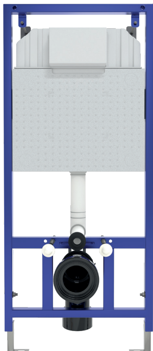
Инсталляция скрытого монтажа NOVUM 525
