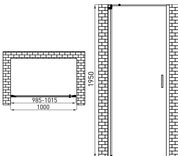
Душевая дверь BERGES LEGOS LS-1 арт 062022
