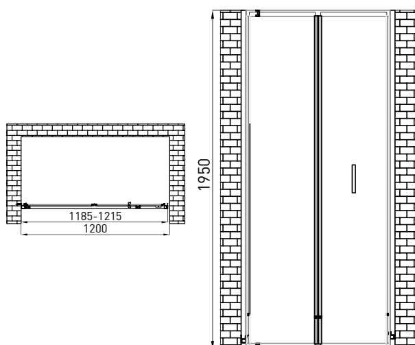
Душевая дверь BERGES LEGOS LS-4 арт 062030
