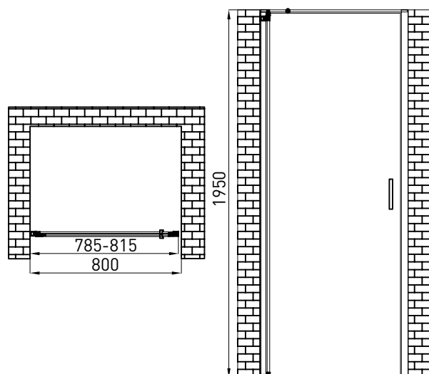
Душевая дверь BERGES LEGOS LS-1 арт 062021
