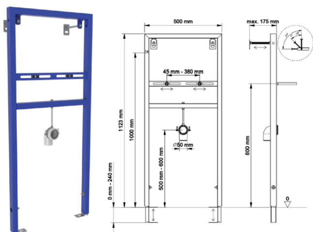
Инсталляция для скрытого монтажа раковины
