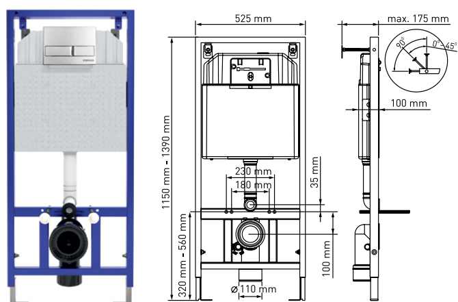
Инсталляция для скрытого монтажа подвесного унитаза
