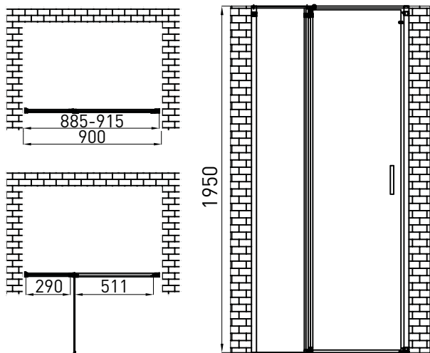
Душевая дверь BERGES LEGOS LS-2 арт 062024
