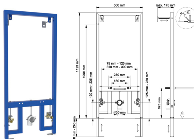
Инсталляция для скрытого монтажа биде
