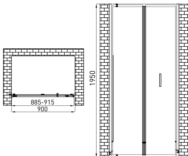
Душевая дверь BERGES LEGOS LS-4 арт 062029
