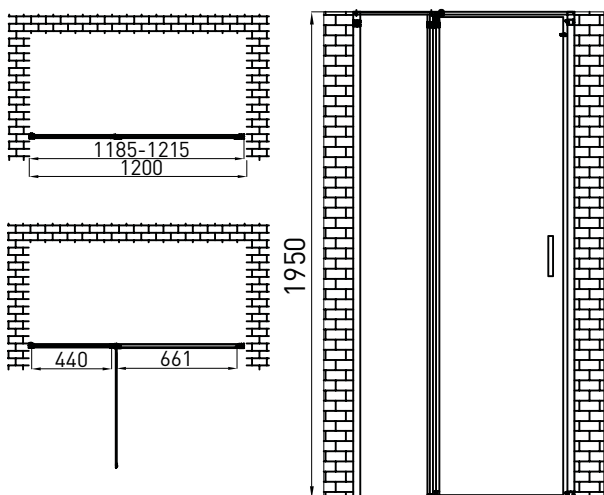
Душевая дверь BERGES LEGOS LS-2 арт 062025
