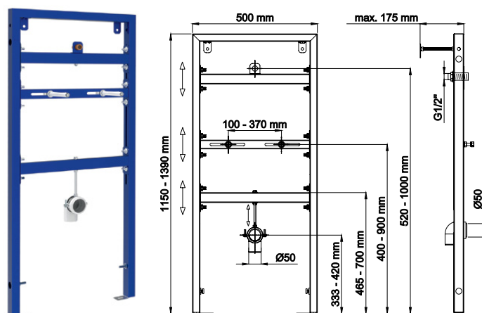
Инсталляция для скрытого монтажа писсуара
